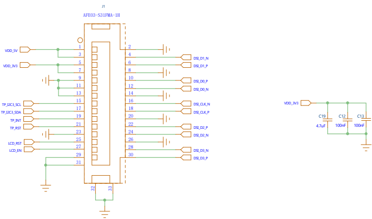
3.5寸(MIPI_LCD 800*480)接口电路
