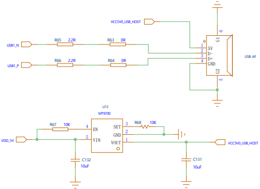
USB接口电路
