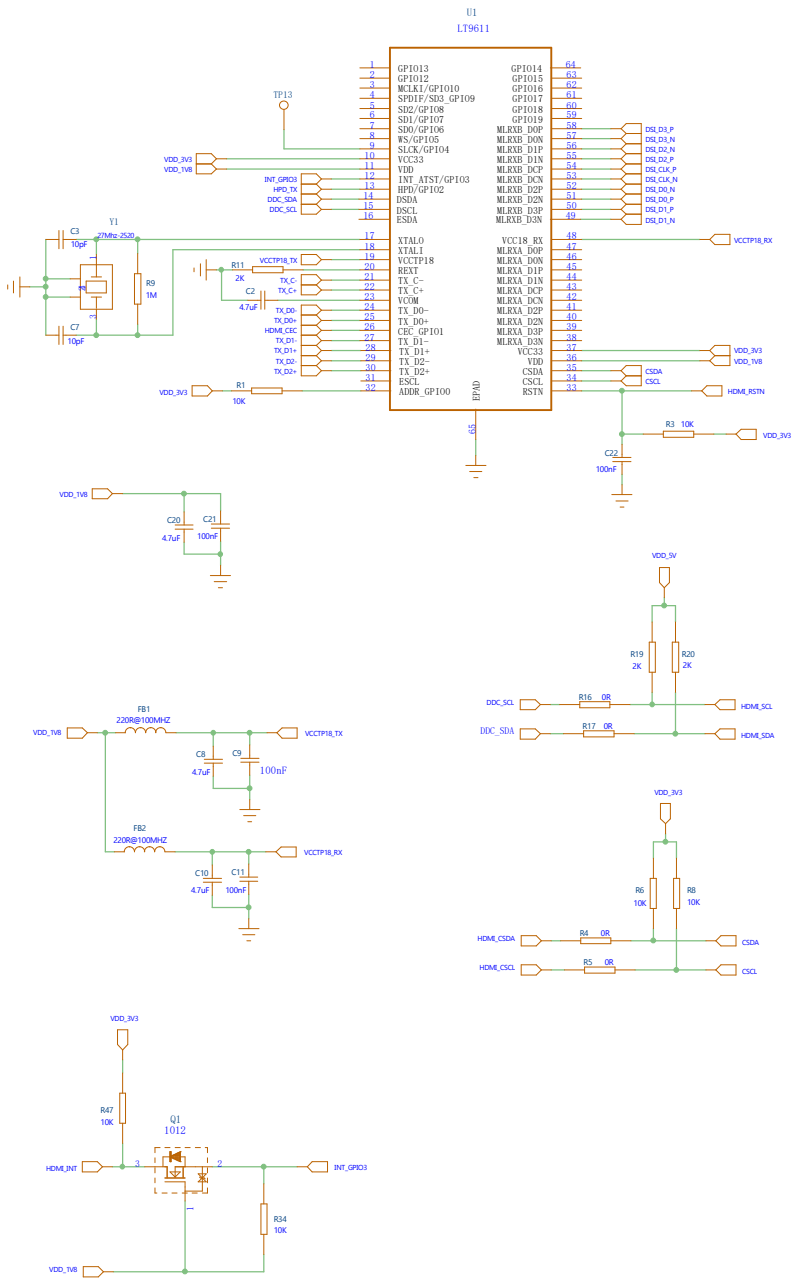
MIPI转HDMI 电路
