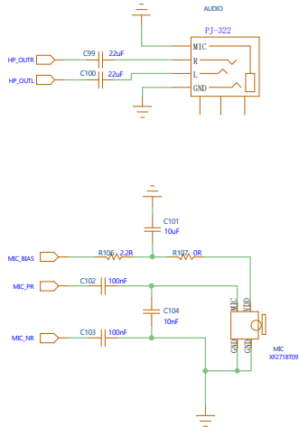
Audio_Jack/MIC电路
