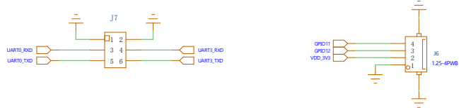
Debug/UART_I2C接口电路
