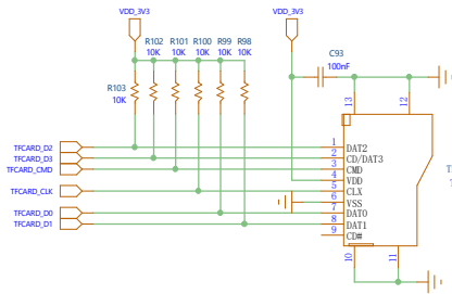
TF Card接口电路
