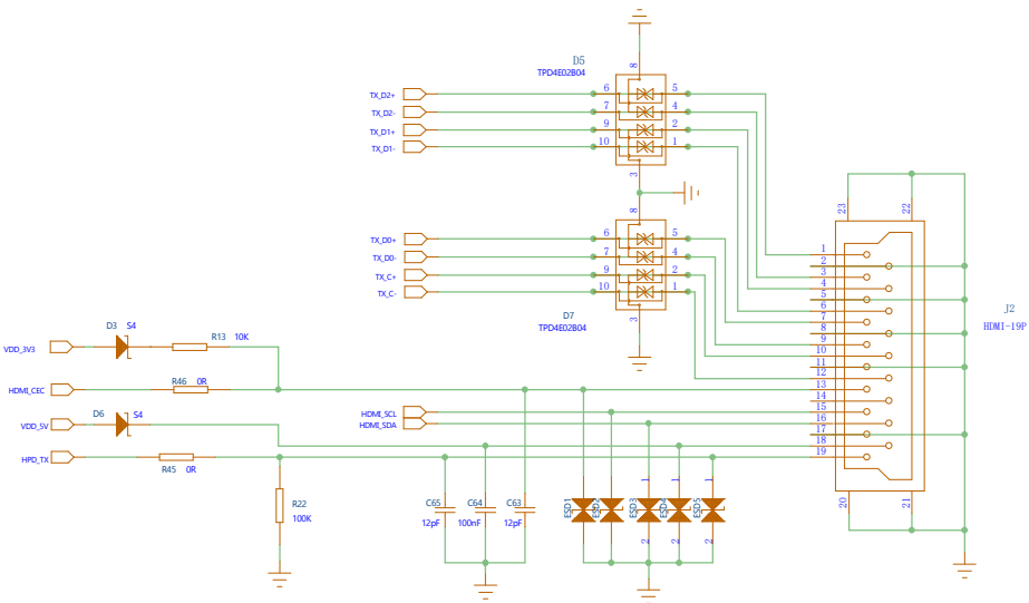
HDMI接口电路
