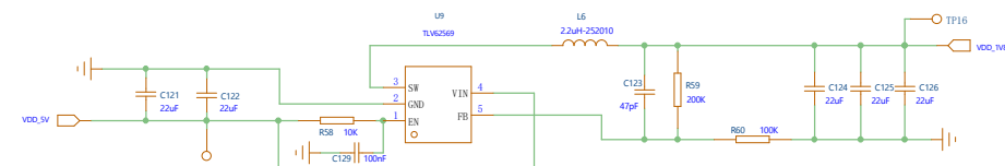
板载4路主电源供电电路
